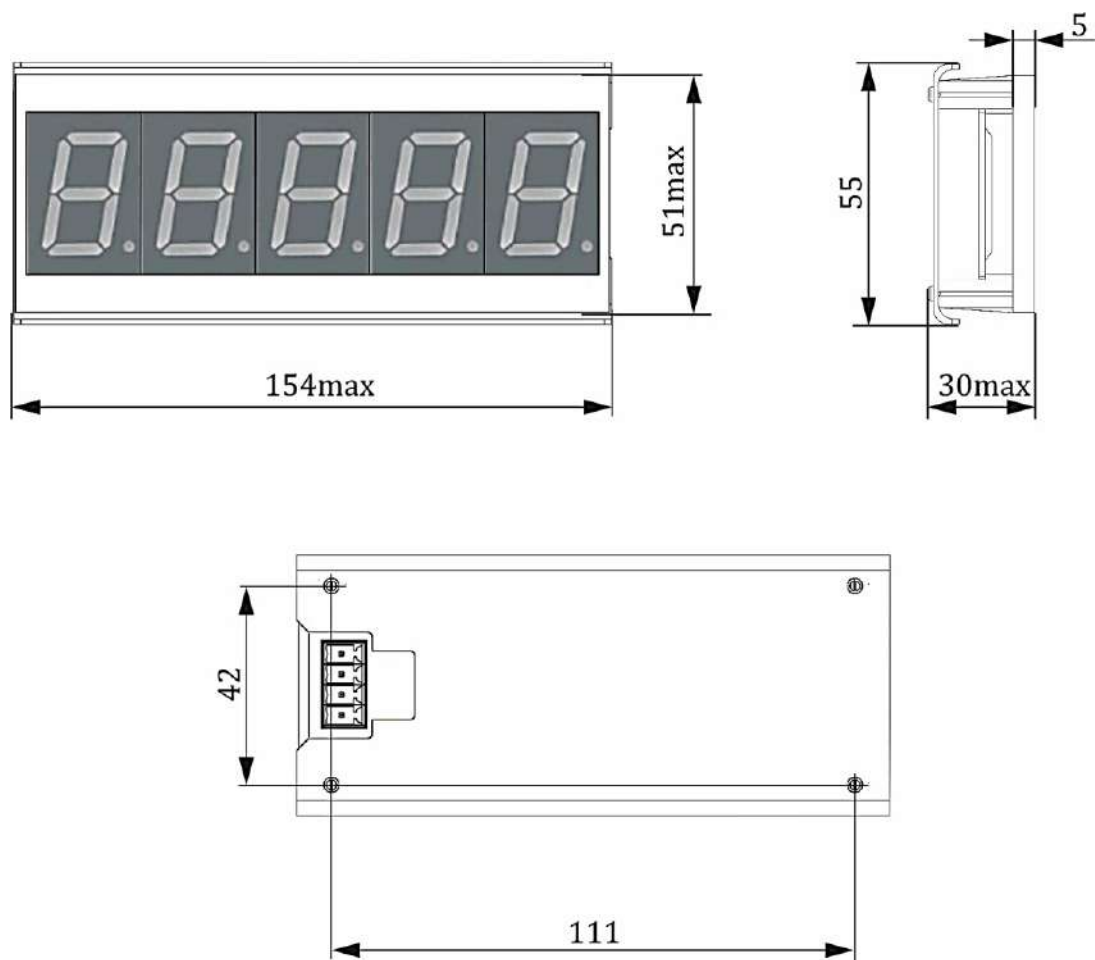
Рисунок Б.5 – Габаритные и установочные размеры внешнего показывающего устройства E8DU
