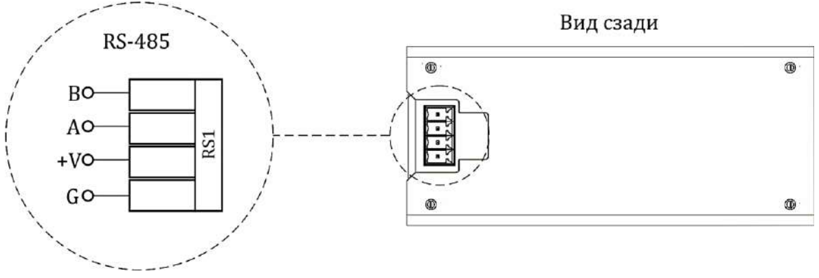
Рисунок Б.10 – Схемы электрические подключения E8DU
