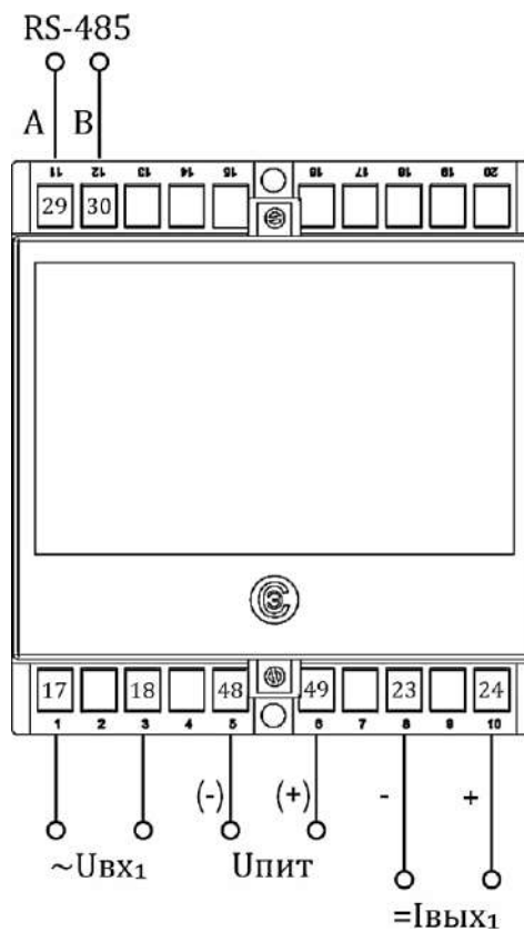
б) Корпус E20 (1 вход, 1 аналоговый выход, 1 порт RS-485)
