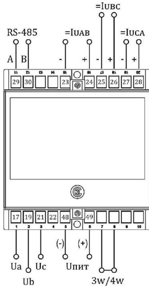
б) Корпус EB20
