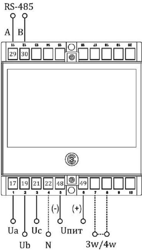
Корпус EB20 (3 входа с объединенной нейтралью, 1 порт RS-485)
