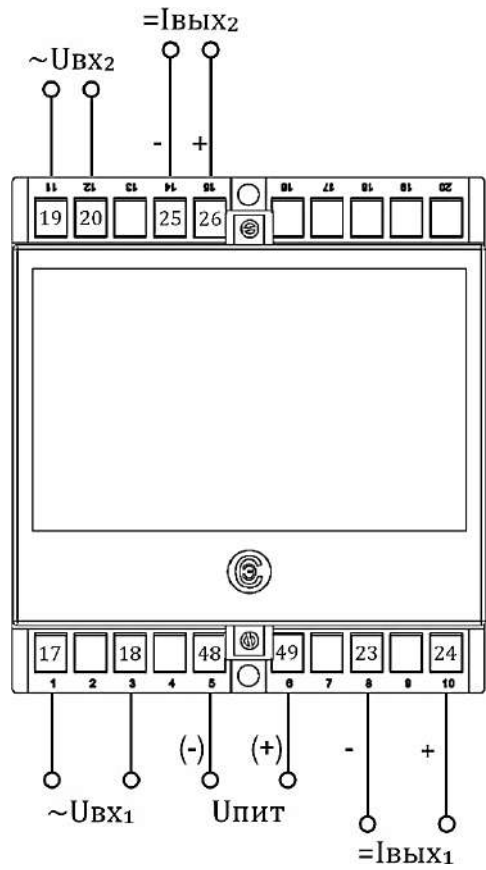
б) Корпус E20 (2 входа, 2 аналоговых выхода)
