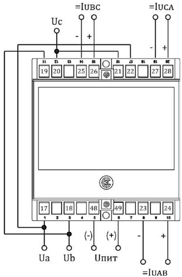
б) Корпус Е20 (3 входа, 3 аналоговых выхода) схема для контроля междуфазных напряжений
